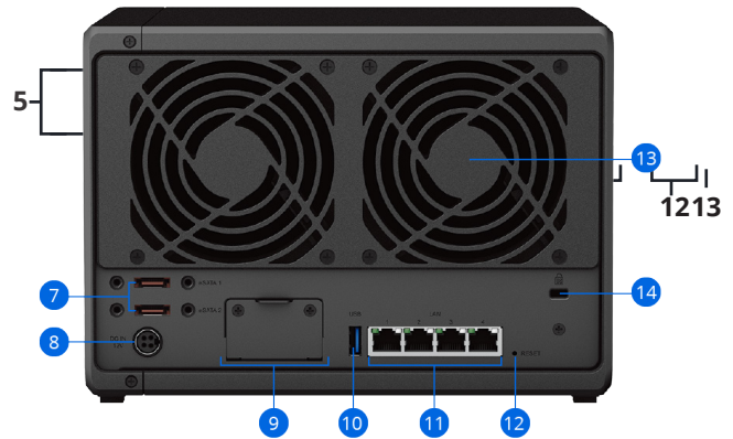
Rückseite
